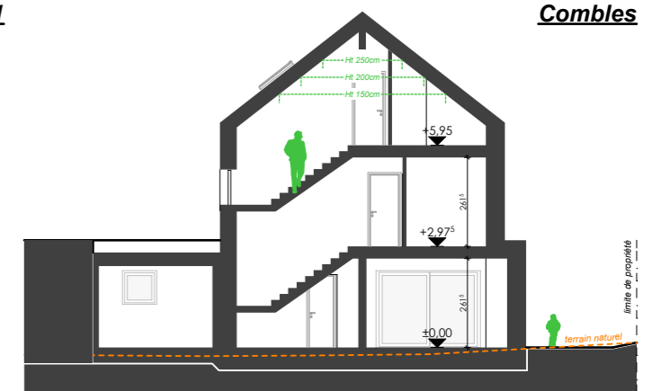
Coupe de principe éch. 1/200
