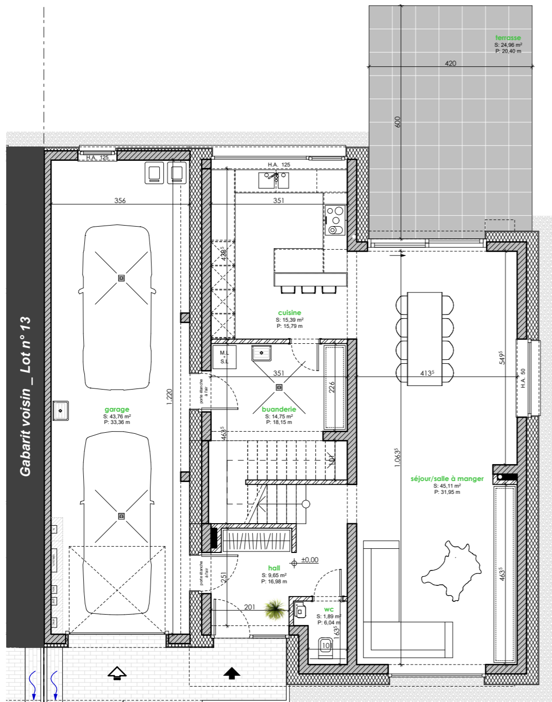
Rez-de-chaussée
